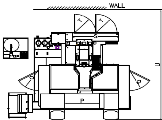
TMQ-13外型尺寸圖
